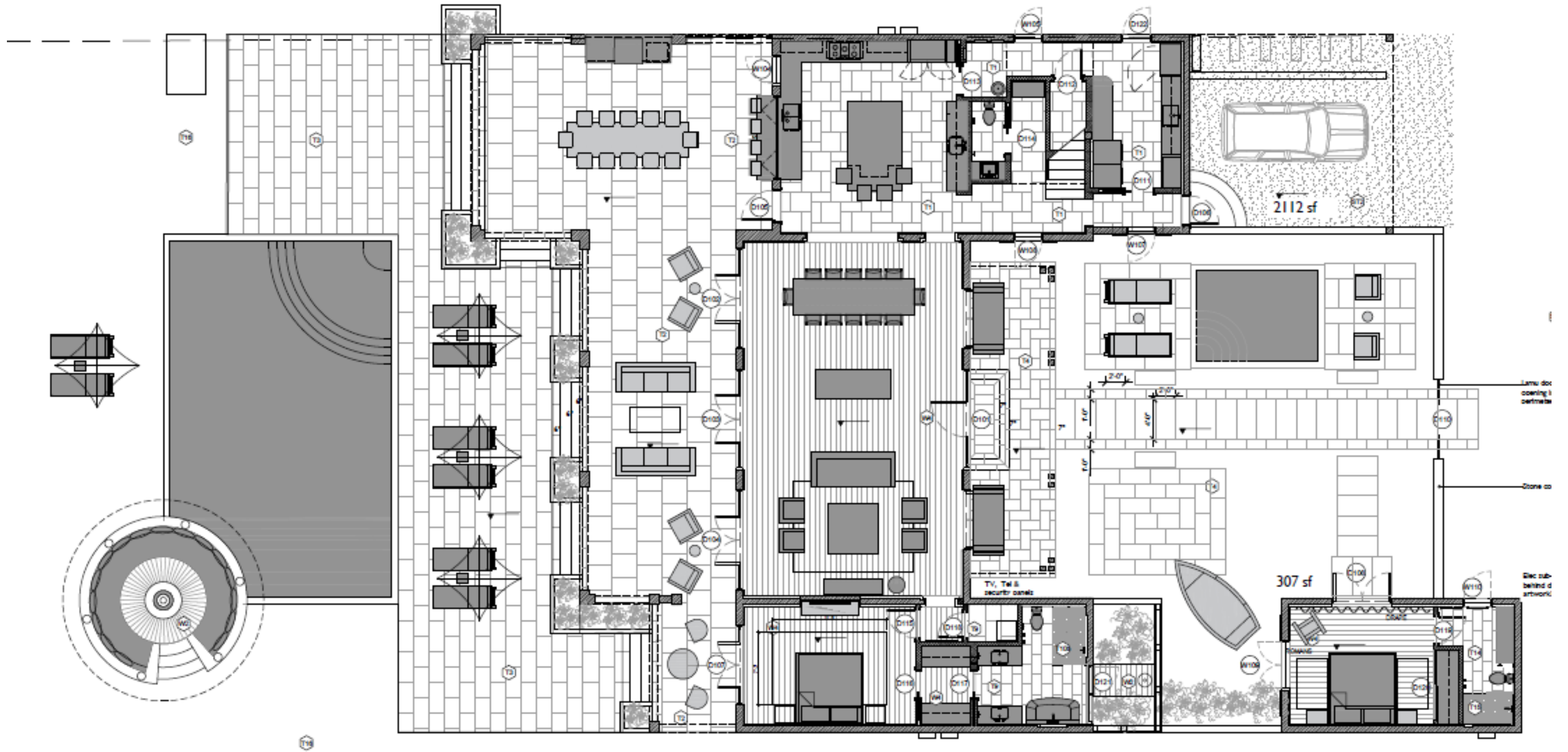
LEVEL 1 - Kisiwa House
