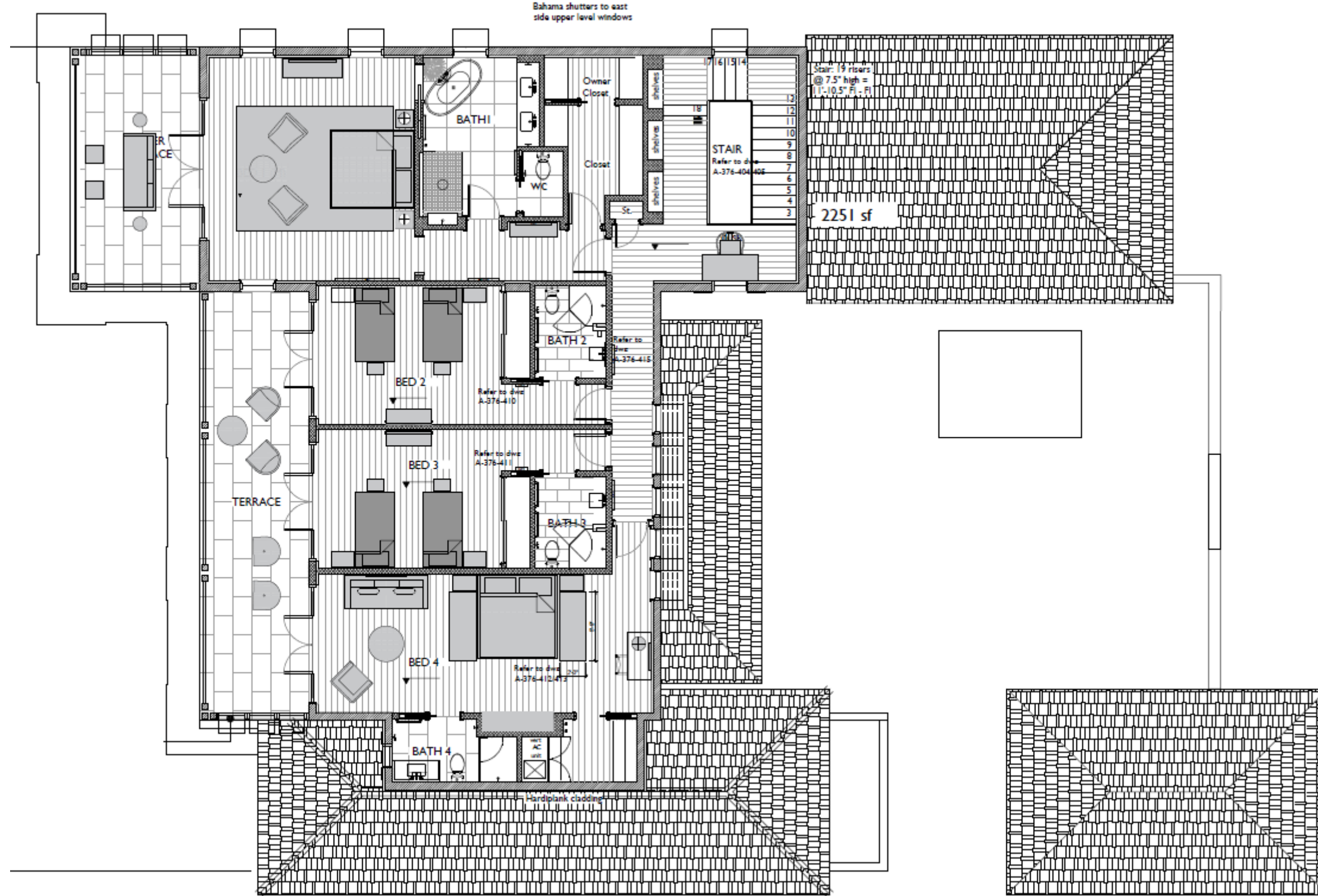
LEVEL 2 - Kisiwa House
